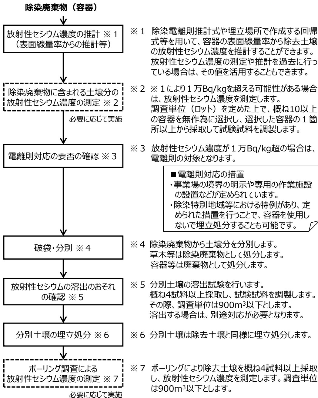
図 5-16 分別土壌の放射性セシウム濃度の把握と埋立処分の流れ
