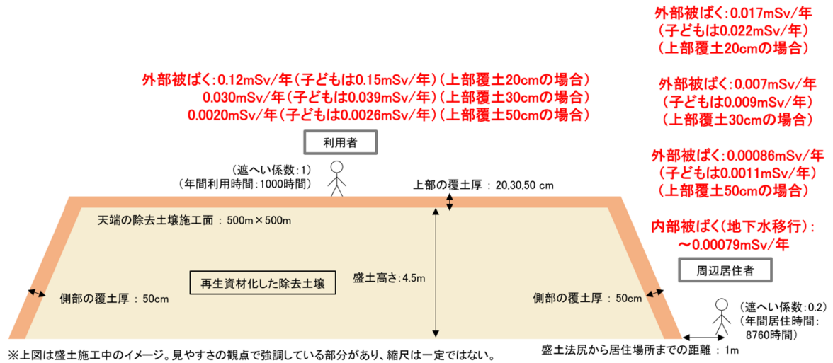
図 2-4 追加被ばく評価計算（維持管理中）の結果
