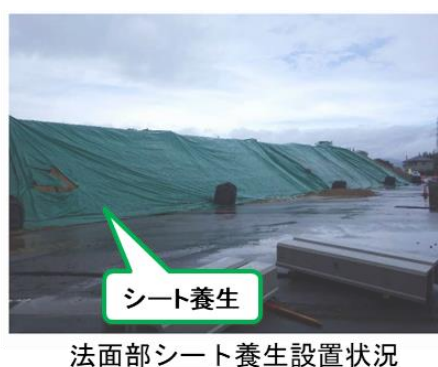
図 2-11 施工中の飛散・流出防止対策の実施例
