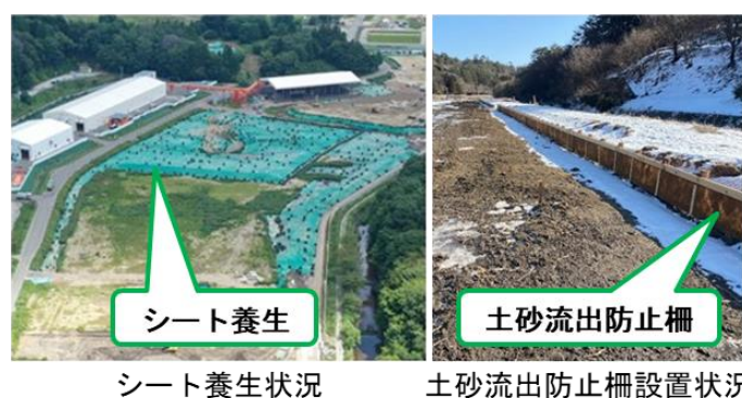
図 2-11 施工中の飛散・流出防止対策の実施例
