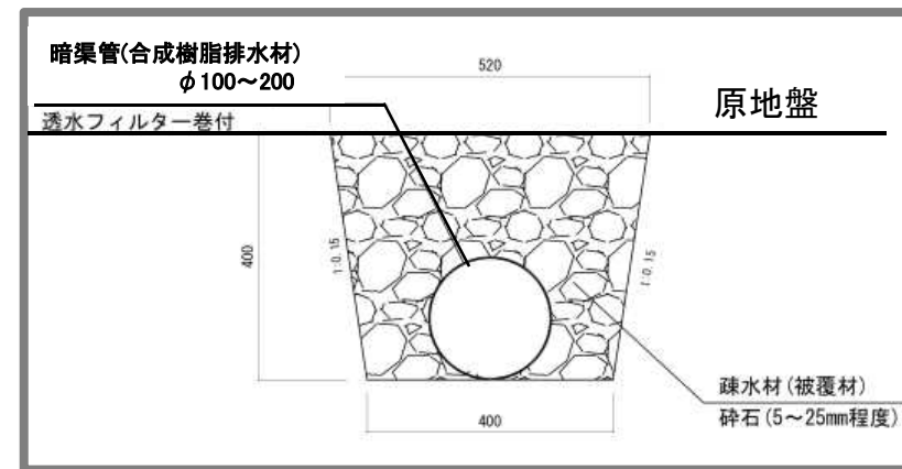
湧水処理構造
