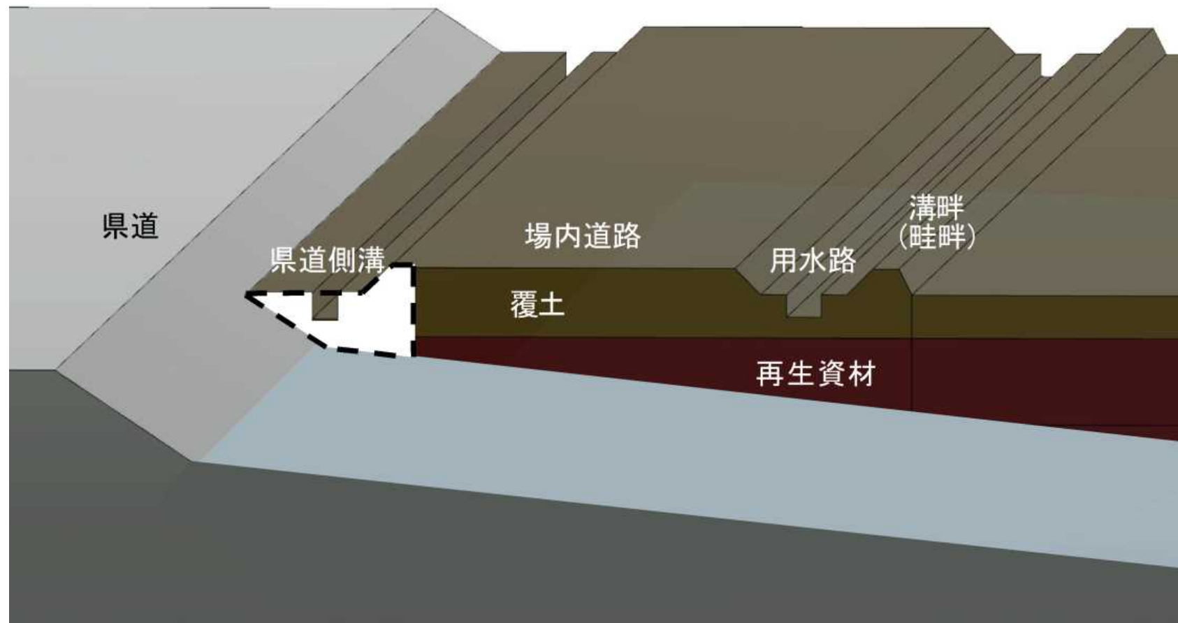
県道側の構造等イメージ図
