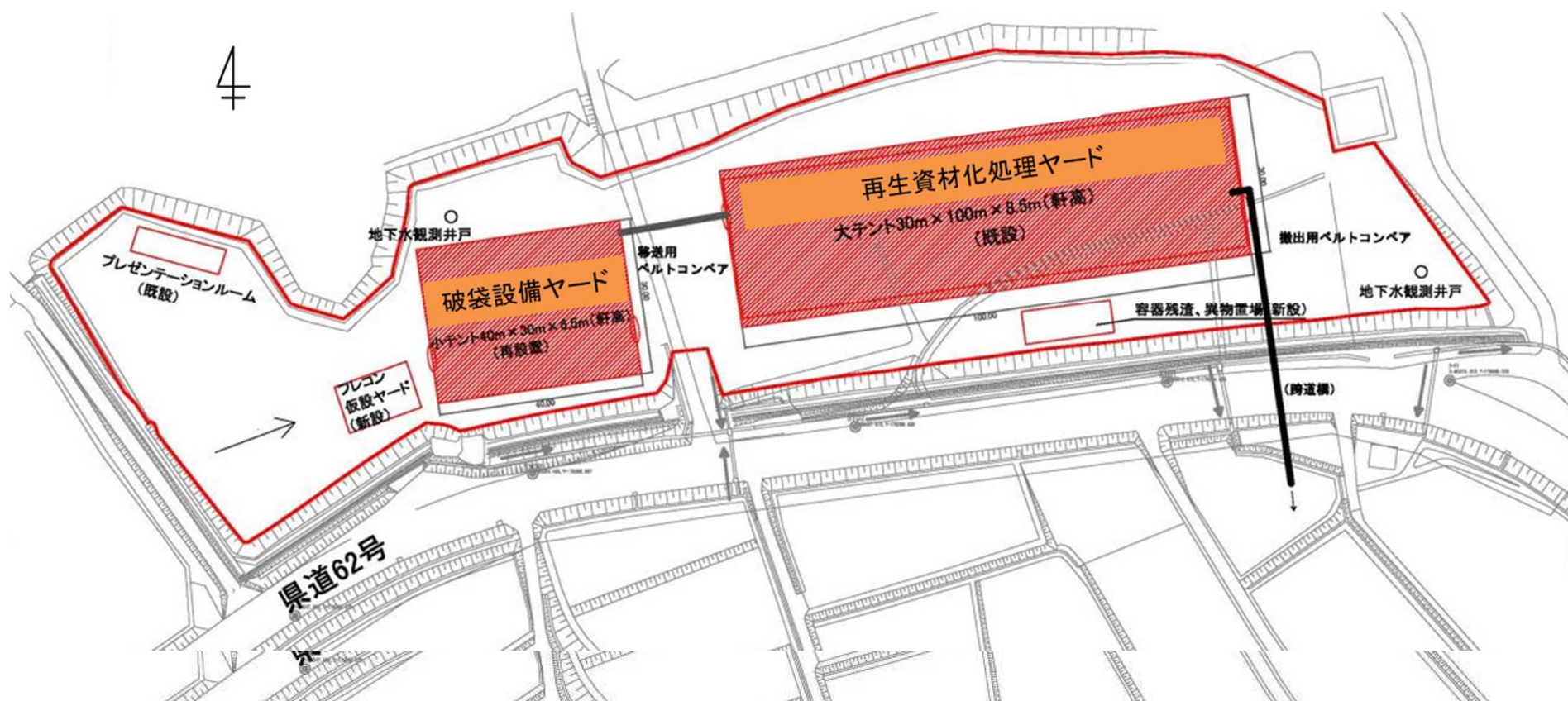
再生資材化施設の概要
