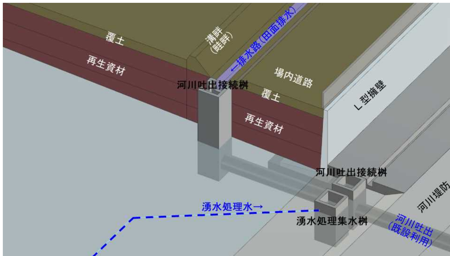
比曽川沿いの構造等イメージ図
