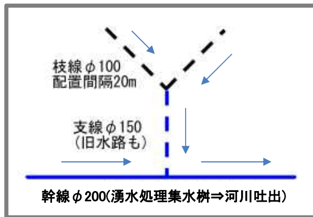
湧水処理平面イメージ
