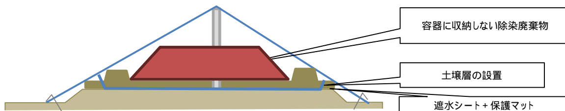
図 2-12 水分を含む除染廃棄物を容器に収納しない場合の汚水流出防止 (例)
